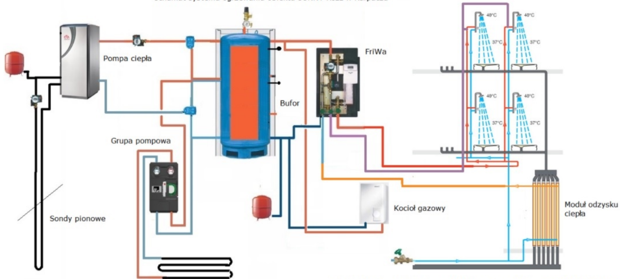
Schemat systemu ogrzewania obiektu SUNNY HILL w Karpaczu
